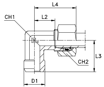
Typ: 1058...4 Ring B4
